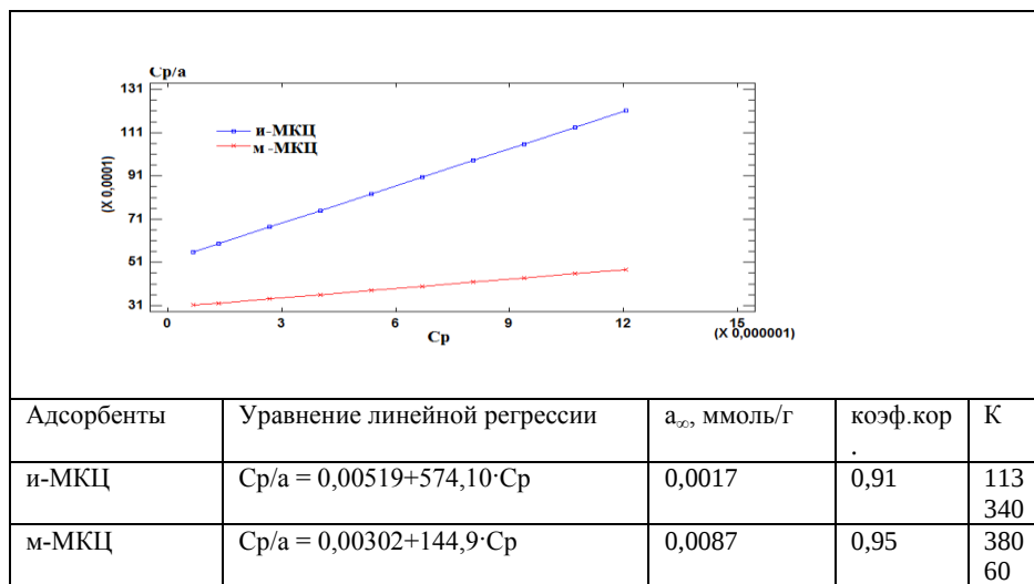
Рис.7 Адсорбция из водных растворов метилового оранжевого на исходном и модифицированном образцах МКЦ в координатах уравнений Ленгмюра
