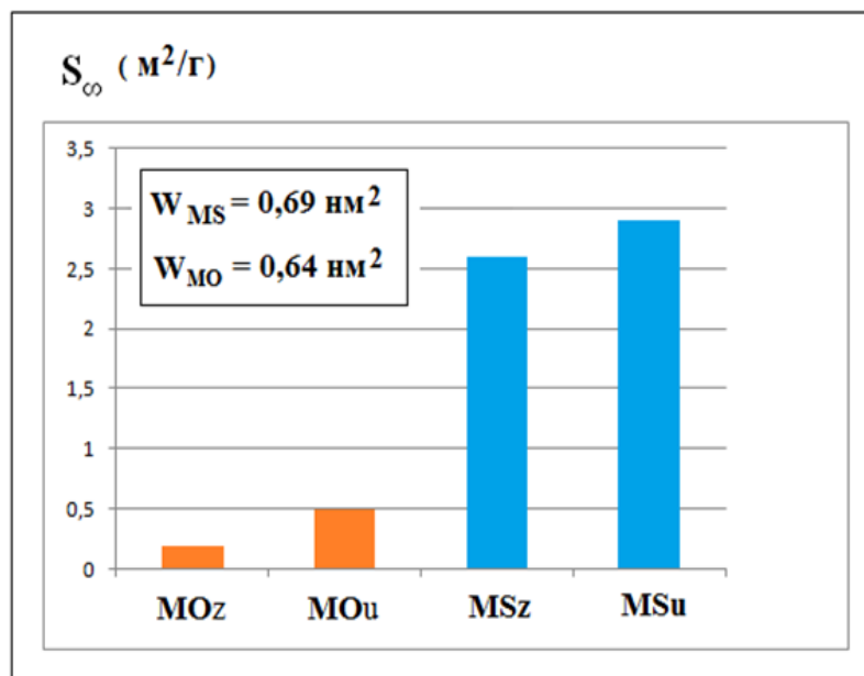
Рис. 3 Пределные значения удельных площадей поверхности адсорбентов по метиленовому синему и метиловому оранжевому
