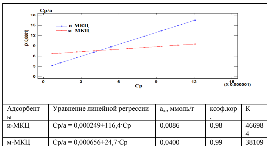
Рис.3. Адсорбция из водных растворов акридинового оранжевого на исходном и модифицированном образцах МКЦ в координатах уравнений Ленгмюра
