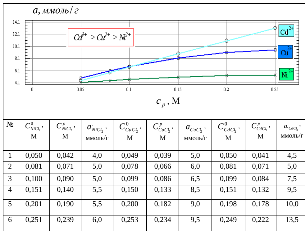
Рис.1 Изотермы адсорбции из водных растворов хлоридов никеля, меди и кадмия на золе угля Кара -Кече, определенные при 298 0 К
