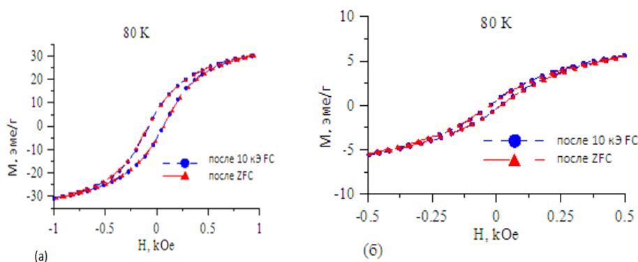
Рис. 2. Кривые гистерезиса магнетита \text{Fe}_3\text{O}_4 - (а), нанокмпозита \text{Fe}_3\text{O}_4 -ГК - (б), полученные при T = 80 К: после охлаждения при H_{\text{ext}} = 10 кЭ и H_{\text{ext}} = 0 кЭ.
