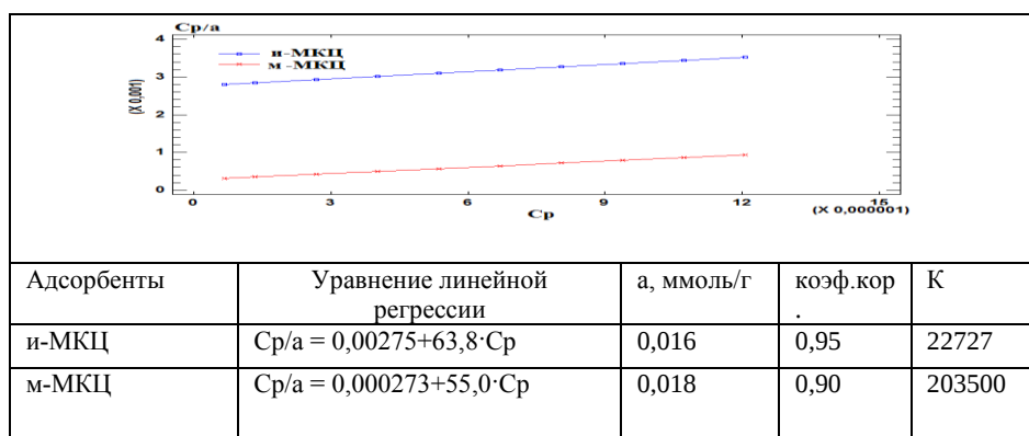
Рис.2 Адсорбция из водных растворов фуксина основного на исходном и модифицированном образцах МКЦ в координатах уравнений Ленгмюра
