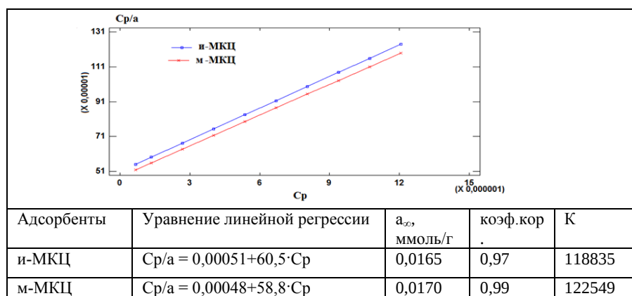
Рис.5 Адсорбция из водных растворов бриллиантового синего на исходном и модифицированном образцах МКЦ в координатах уравнений Ленгмюра
