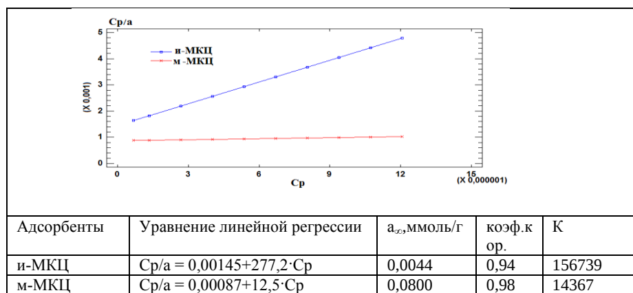
Рис.6 Адсорбция из водных растворов эозина-н на исходном и модифицированном образцах МКЦ в координатах уравнений Ленгмюра
