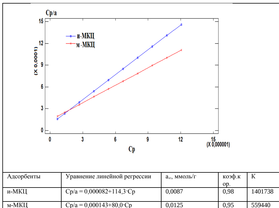
Рис.1 Адсорбция из водных растворов метиленового фиолетового на исходном и модифицированном образцах МКЦ в координатах уравнений Ленгмюра
