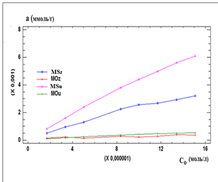
Рис.1 Изотермы адсорбции метиленового синего(MS) и метилового оранжевого(MO) на золе(z) и угле (u) Кара- Кече
