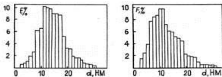
Рис.1. Нормированные гистограммы распределения частиц по размерам
