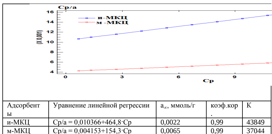
Рис.4. Адсорбция из водных растворов ализаринового желтого на исходном и модифицированном образцах МКЦ в координатах уравнений Ленгмюра
