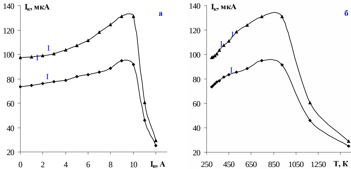
Рис. 2. Зависимость тока коронного разряда положительной (I) и отрицательной (II) полярности от тока нагрева (а) и температуры (б) коронирующего электрода.
