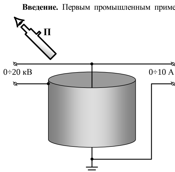
Рис. 1. Разрядная ячейка, реализованная по коаксиальной схеме. П - пирометр регистрирующий температуру коронирующего провода.
