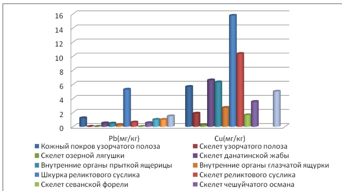
Рис. 6. Содержание тяжёлых металлов в органах животных
