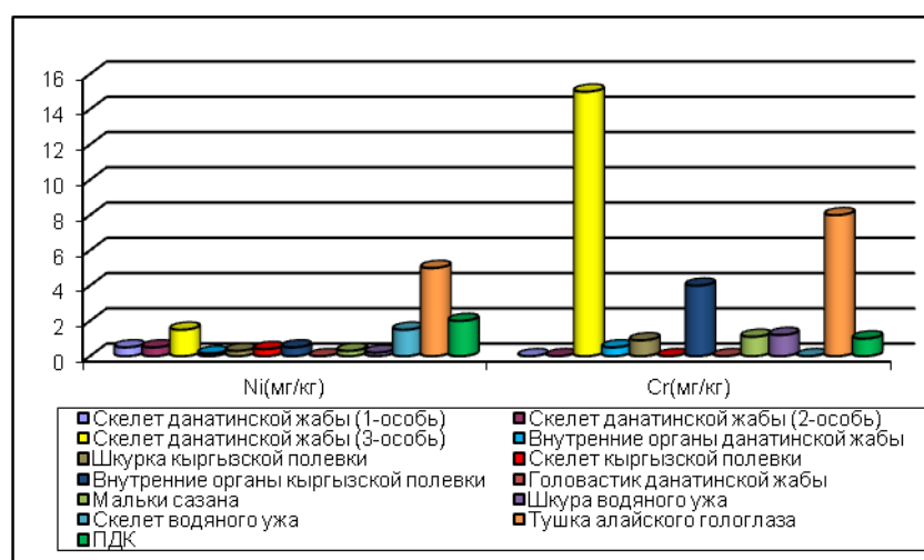
Рис. 17 Содержание химических элементов в органах животных (п.г.т. Ак-Тюз)
