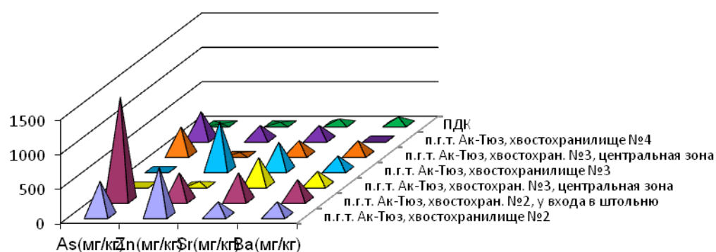
Рис. 2 Содержание химических элементов в почвенных образцах(п.г.т. Ак-Тюз)
