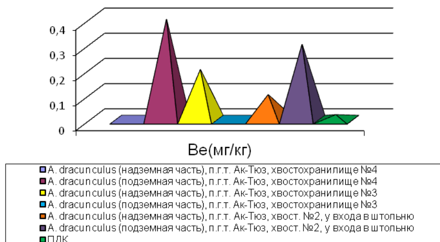
Рис. 9Содержание химических элементов в растениях (п.г.т. Ак-Тюз)
