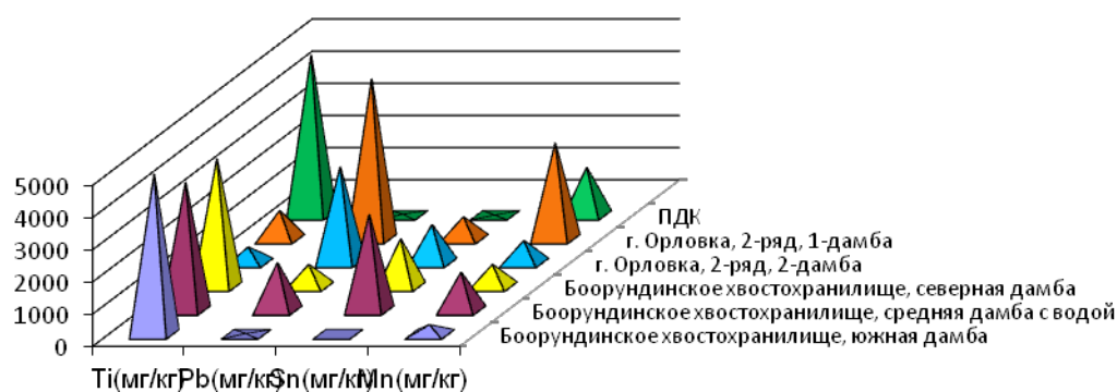
Рис. 4 Содержание химических элементов в почвенных образцах (г. Орловка и с. Боорундинское)
