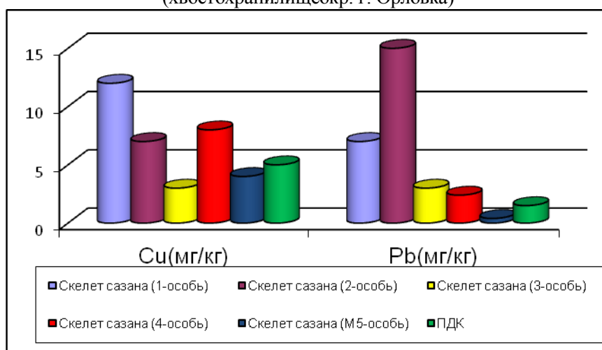
Рис. 20 Содержание химических элементов в органах животных (хвостохранилищеокр. г. Орловка)
