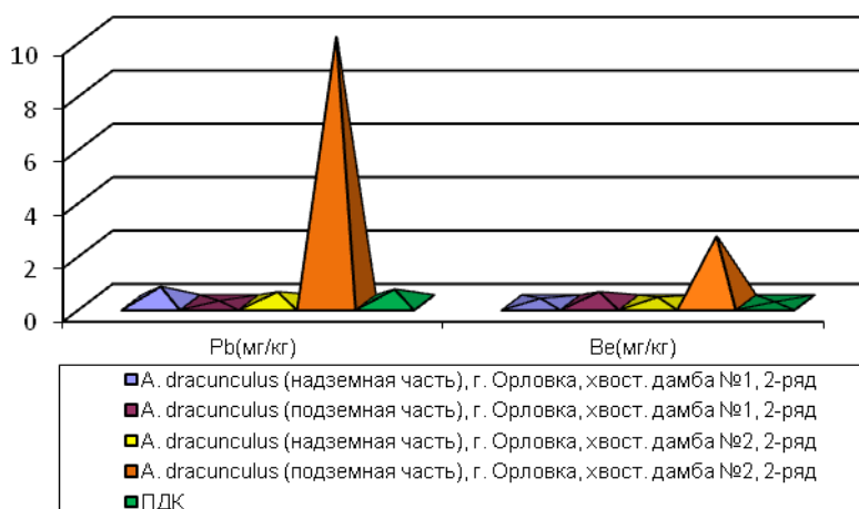
Рис. 15 Содержание химических элементов в растениях (г. Орловка, дамбы около прудов)
