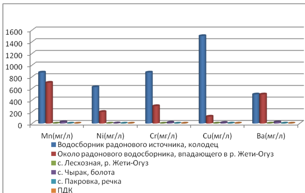
Рис.4. Содержание химических элементов в пробах воды (Джети-Огуз)
