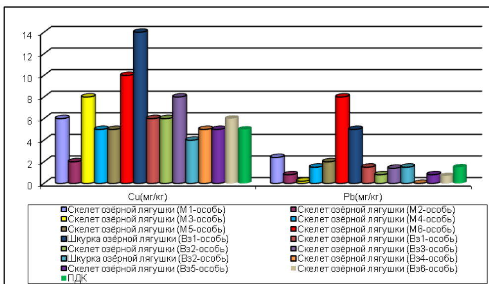
Рис. 18 Содержание химических элементов в органах животных
