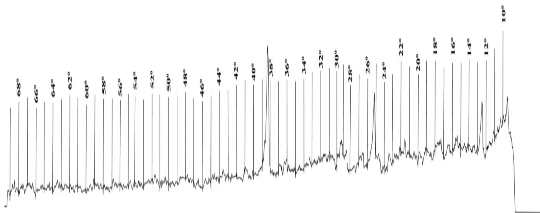
Рис.3 Дифрактограмма \text{FeCl}_3 \cdot 3 \text{NH}_2\text{C}_6\text{H}_4\text{COOH} Рентгенографический анализ \text{FeCl}_3 - \text{NH}_2\text{C}_6\text{H}_4\text{COOH} - \text{H}_2\text{O}(\text{C}_2\text{H}_5\text{OH})
