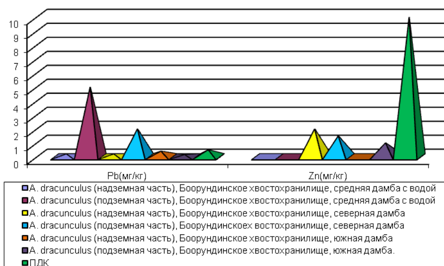
Рис. 11 Содержание химических элементов в растениях (с. Боорундинское)
