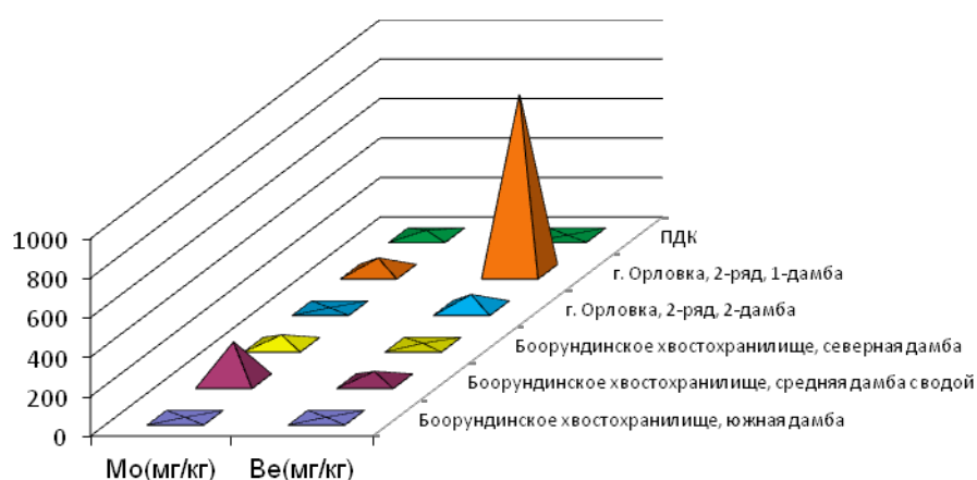
Рис. 6. Содержание химических элементов в почвенных образцах (г. Орловка и с. Боорундинское)
