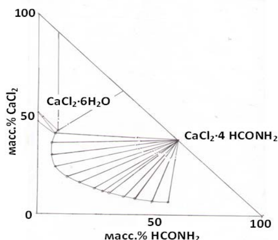
Рис. 1. Изотерма растворимости системы \text{CaCl}_2 - \text{HCONH}_2 - \text{H}_2\text{O} при 298K
