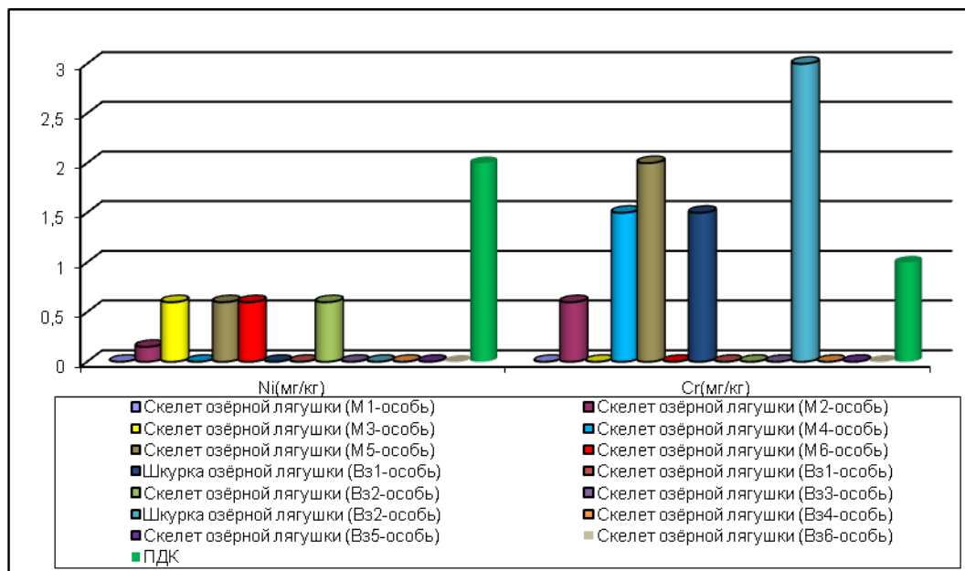
Рис. 19 Содержание химических элементов в органах животных (хвостохранилищеокр. г. Орловка)
