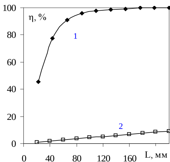
Рис.4. Зависимость степени улавливания порошка кремния от длины электрофилтра. 1-эксперимент 2-расчет.
