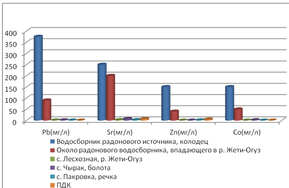
Рис.5. Содержание химических элементов в пробах воды (Джети-Огуз)
