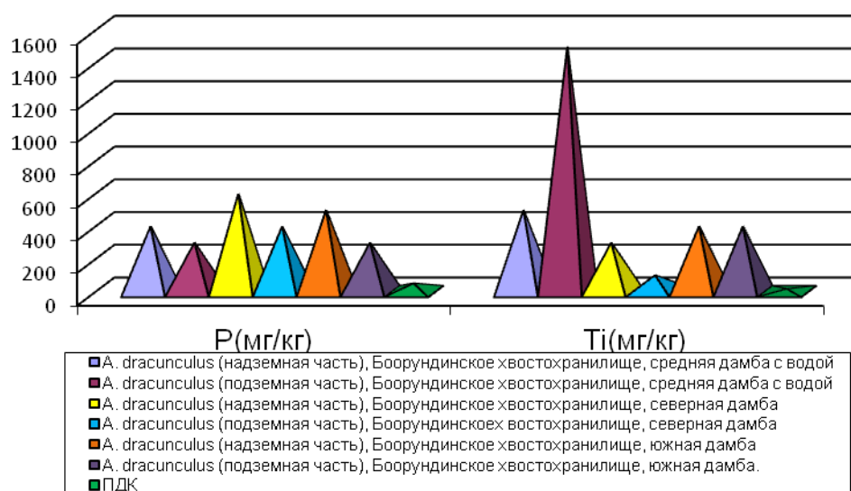
Рис. 13 Содержание химических элементов в растениях (с. Боорундинское)
