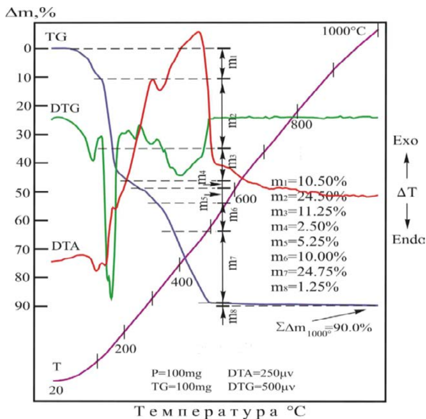
Рис.2. Дериватограмма \text{FeCl}_3 \cdot 3\text{NH}_2\text{C}_6\text{H}_4\text{COOH}
