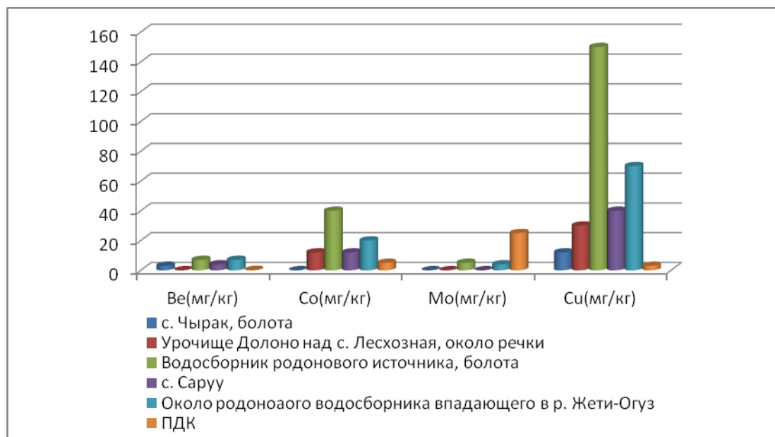
Рис.3. Содержание химических элементов в почвенных образцах (р-н.Джети-Огуз)
