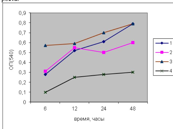
Диагр.1. Степень аккумулятивных способностей высоких концентраций свинца культурами Bacillus megatherium , Bacillus cereus (H5-8 + H5-2).
