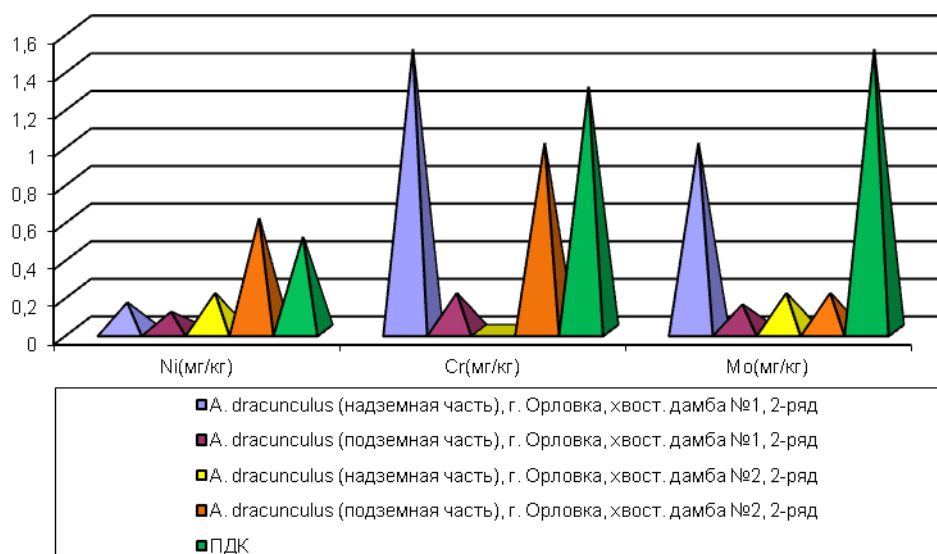
Рис. 14 Содержание химических элементов в растениях (г. Орловка, дамбы около прудов)
