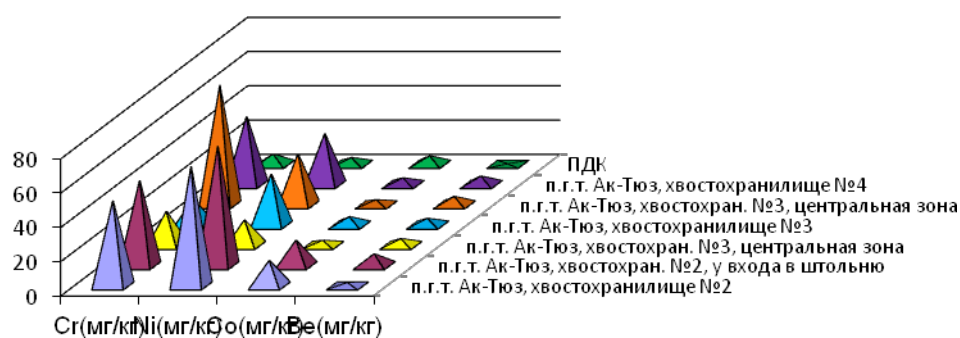
Рис. 3 Содержание химических элементов в почвенных образцах (п.г.т. Ак-Тюз)
