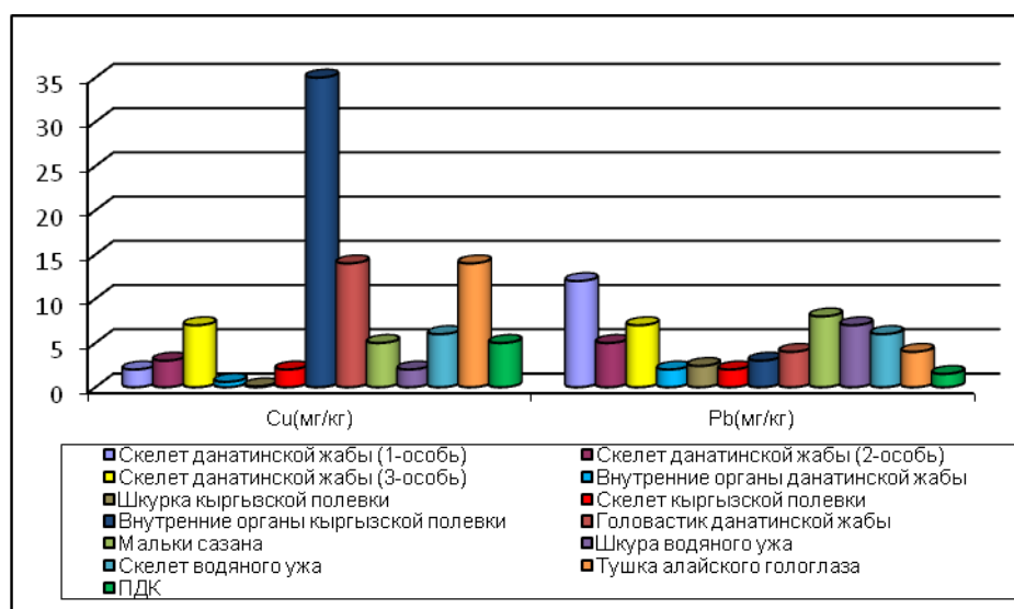
Рис. 16 Содержание химических элементов в органах животных (п.г.т. Ак-Тюз)
