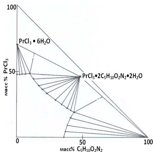
Рис. 1. Диаграмма растворимости системы PrCl 3 – C 5 H 10 O 2 N 2 – H 2 O при 298K
