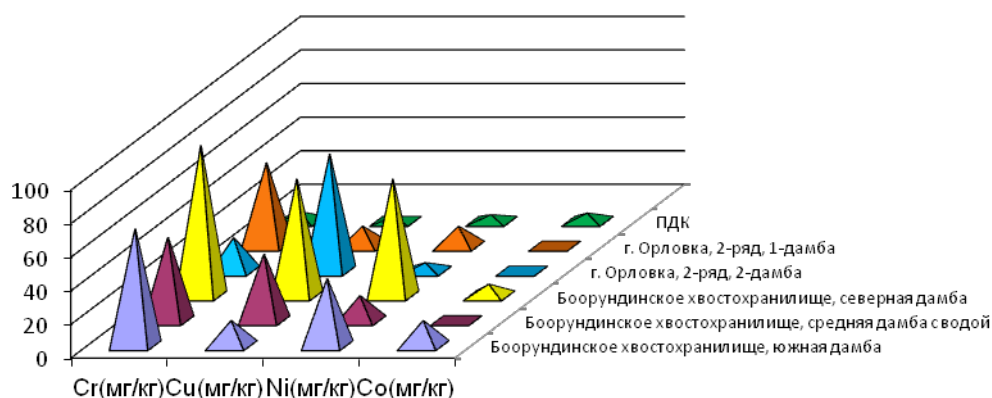
Рис. 5. Содержание химических элементов в почвенных образцах (г. Орловка и с. Боорундинское)
