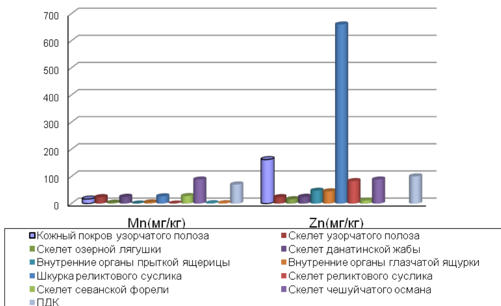
Рис. 7. Содержание тяжёлых металлов в органах животных
