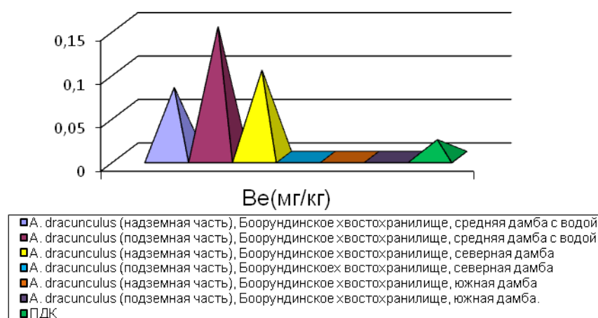
Рис. 12 Содержание химических элементов в растениях (с. Боорундинское)
