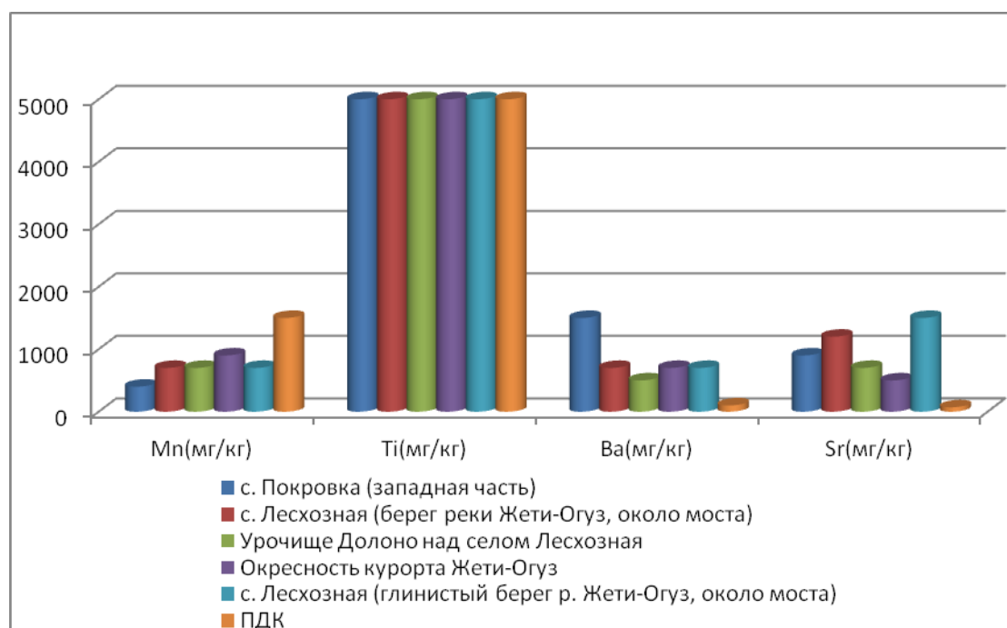
Рис.1. Содержание химических элементов в почвенных образцах (р-н.Джети-Огуз)
