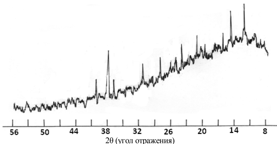
Рис.2. Дифрактограмма соединения \text{PrCl}_3 \cdot 2\text{C}_5\text{H}_{10}\text{O}_2\text{N}_2 \cdot 2\text{H}_2\text{O}
