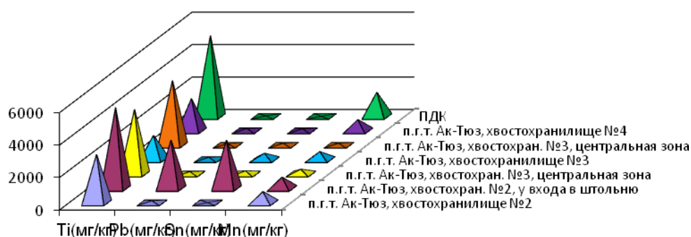
Рис. 1 Содержание химических элементов в почвенных образцах (п.г.т. Ак-Тюз)
