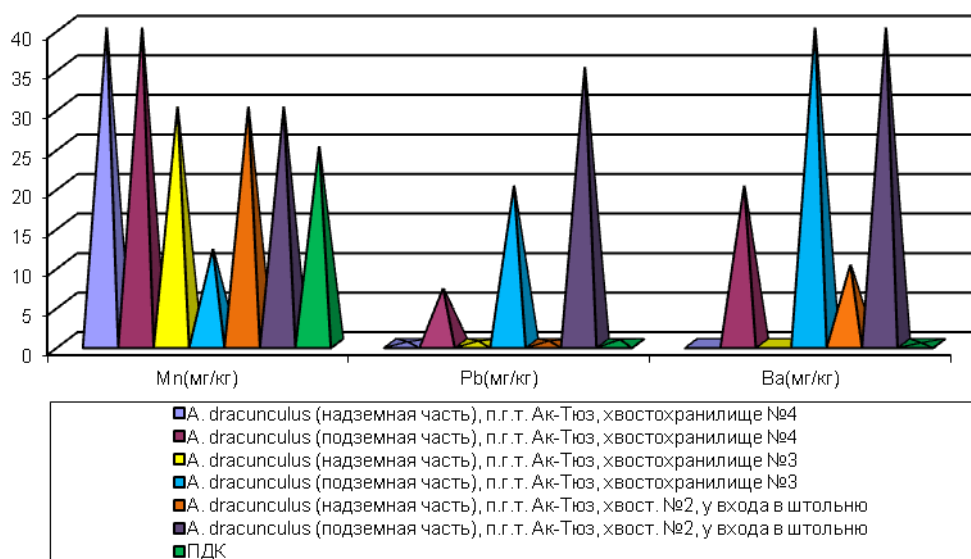
Рис. 8 Содержание химических элементов в растениях (п.г.т. Ак-Тюз)
