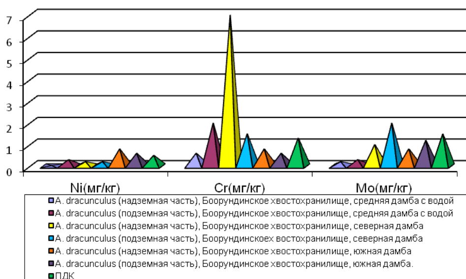
Рис. 10Содержание химических элементов в растениях (с. Боорундинское)
