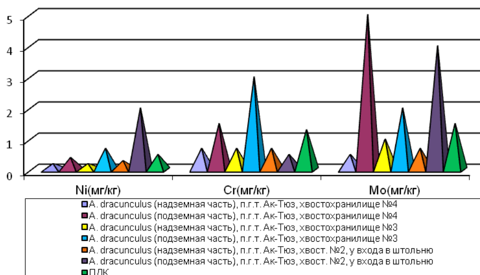
Рис. 7 Содержание химических элементов в растениях (п.г.т. Ак-Тюз)
