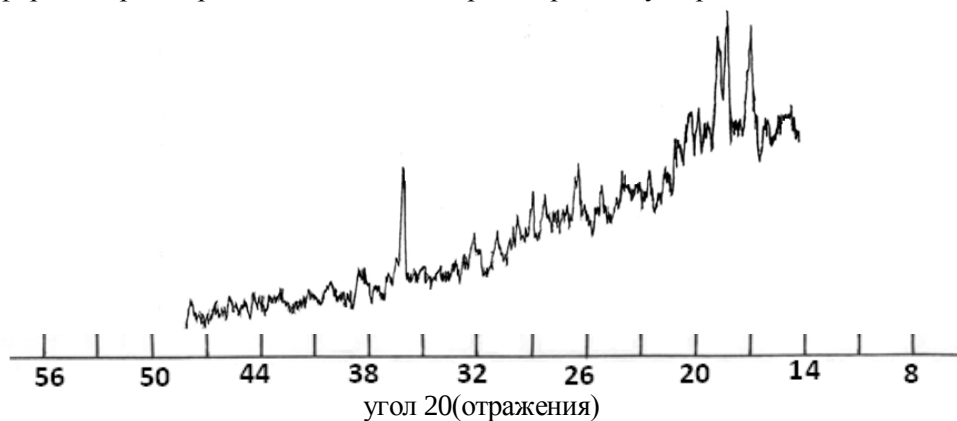
Рис.2. Дифрактограмма соединения \text{Er}(\text{NO}_3)_3 \cdot 2\text{C}_5\text{H}_{10}\text{O}_2\text{N}_2 \cdot 2\text{H}_2\text{O}
